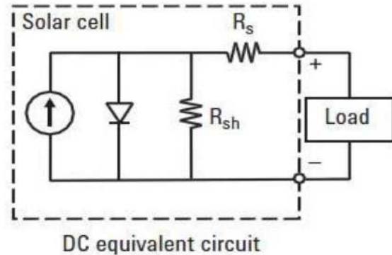
Fig. 3 D.C Equivalent Circuit.
